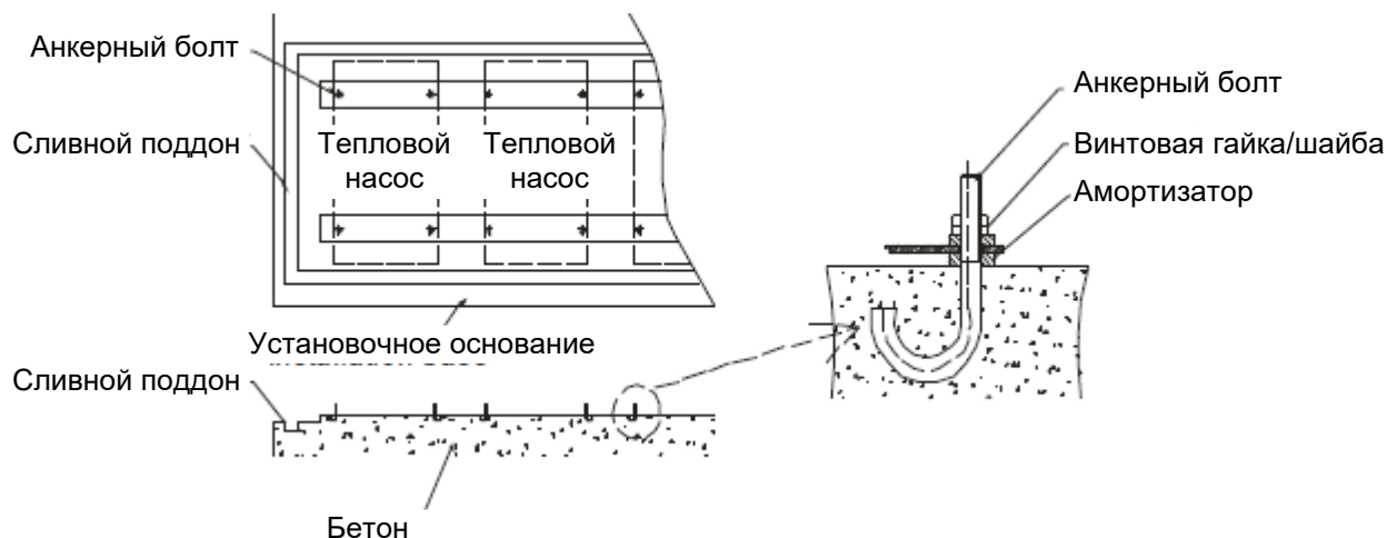
Рисунок 4. Установочное основание
